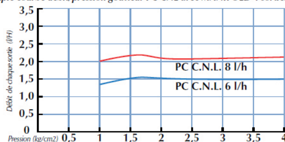
Exemple courbe débit/pression goutteur PC CNL avec MANIFOLD 4 sorties
